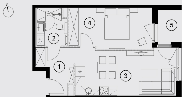
RZUT MIESZKANIA MA29
