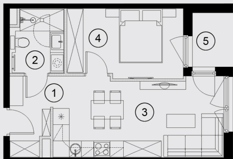
RZUT MIESZKANIA MA30
