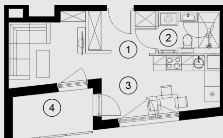
RZUT MIESZKANIA MA35
