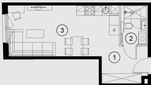
RZUT MIESZKANIA MB13
