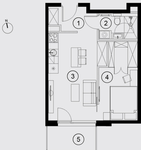
RZUT MIESZKANIA MC04
